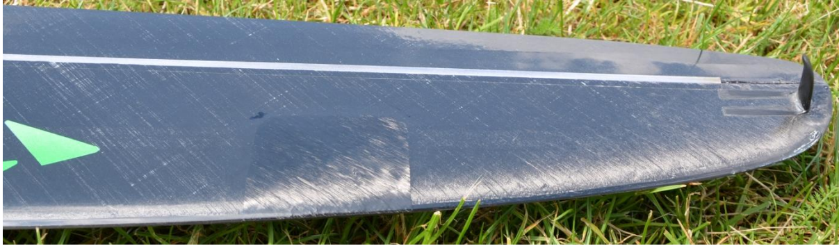
Flügel Feldreparatur
